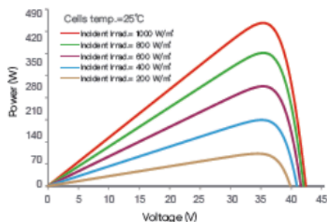
Krzywa prąd-napięcie i moc-napięcie (SL5M108)
